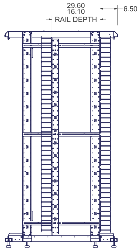
SECTION A-A
