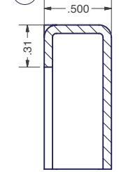
SECTION C-C TYP 4 SIDES
