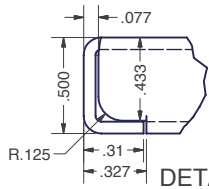
DETAIL A TYP 4 CORNERS
