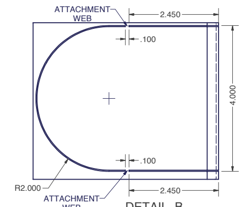
DETAIL B TYP 2 PLACES
